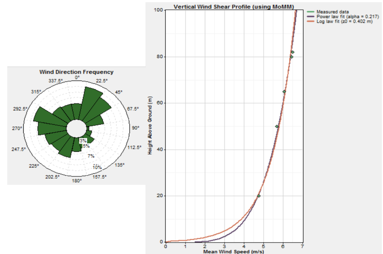
Figure 1 : Rose des vents (source : BORALEX, 2018)
